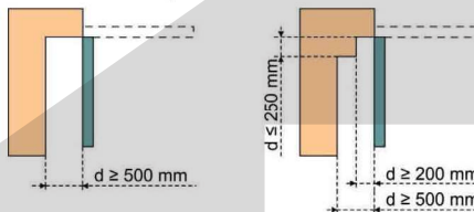
Obrázek 2 – Mechanická ochrana
